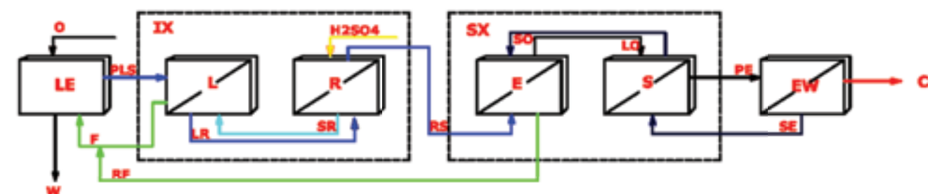
Технолошка шема на процесот L-IX-SX-EW;
